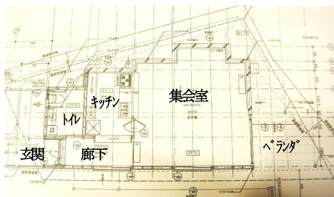
↑ 建物平面図(間取り図)
